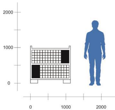
Deutsche Bahn Box (DB) Inhalt ca. 0,75 m 3 ca. 0,80m x 1,08m x 1,20m (L x H x B)
